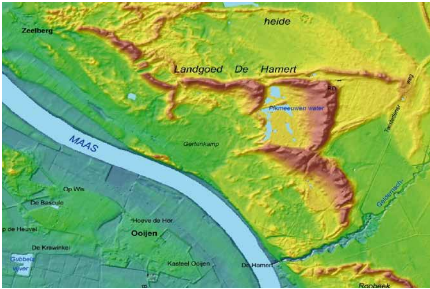
Hoogtekaart van de rivierduinen bij De Hamert, met duidelijk zichtbaar de typische paraboolvorm. Bron: www.ahn.nl
